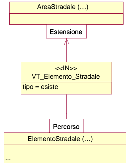
Diagramma 6.1 – Esempio di vincolo topologico esistenziale
