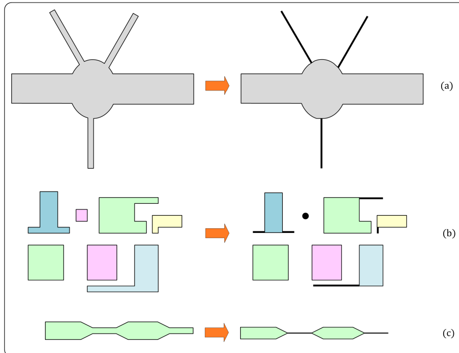
Figura 7.2: Alcuni esempi di collassamenti ammessi.
